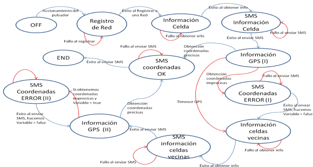
Figura 3.6: Diagrama de estados asociado al funcionamiento del programa.
