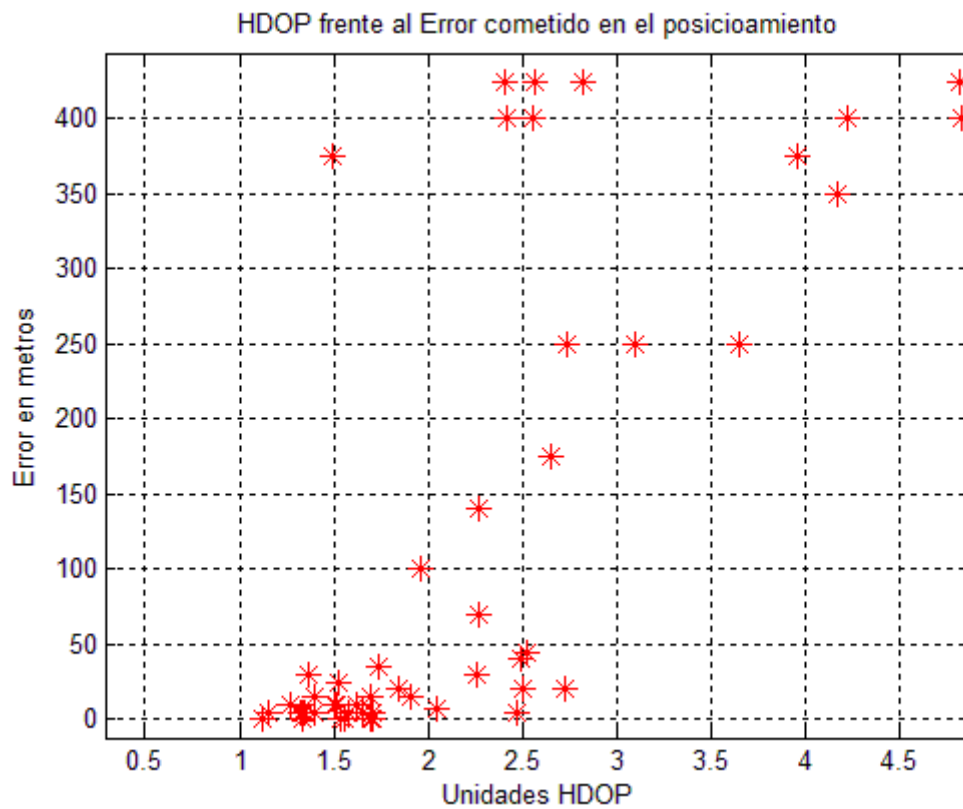
Figura 3.9: Gráfica II con el valor del error en el posicionamiento GPS frente al HDOP.
