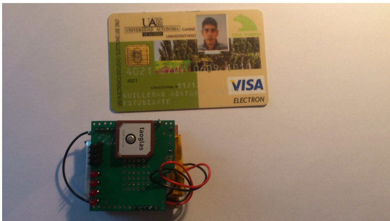
Figura 4.48: Vista superior del dispositivo final de usuario.
