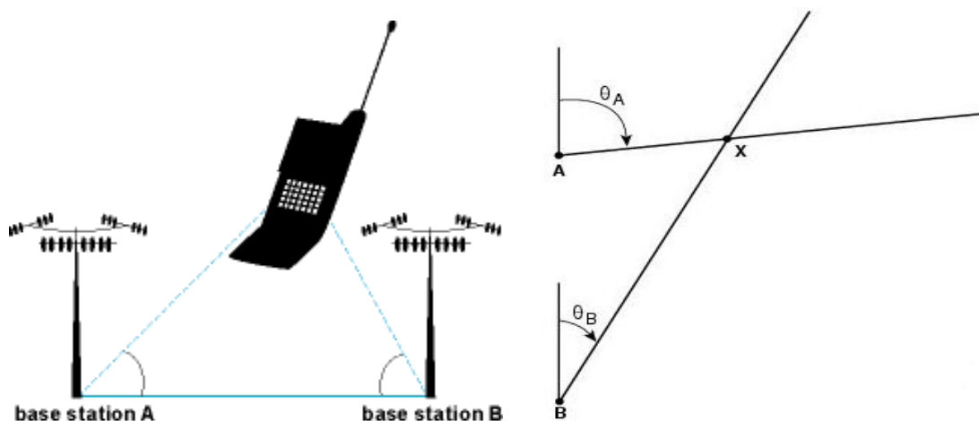
Figura 2.5: Esquema del cálculo del posicionamiento mediante AoA.
