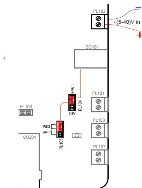
Figura 4.3: Opción escogida para alimentación del EVK2 y su respectiva configuración de jumpers.
