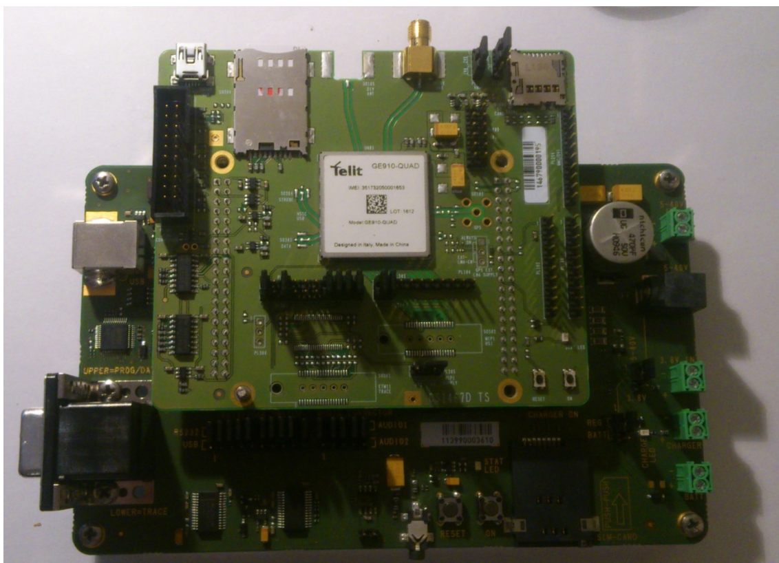
Figura 4.2: EVK2 con la placa interfaz GE910 montada.
