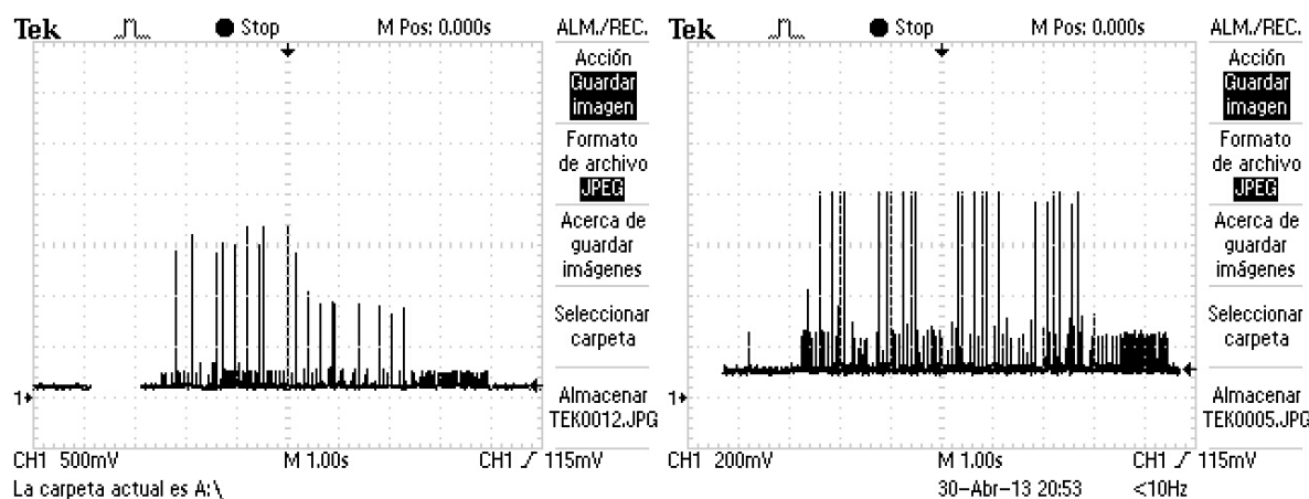
Figura 3.21: Forma de onda osciloscopio para 2 realizaciones diferentes del envío de un SMS.
