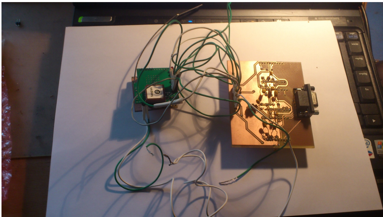
Figura 4.50: Conexión del dispositivo final de usuario con la placa de comunicaciones con el PC.
