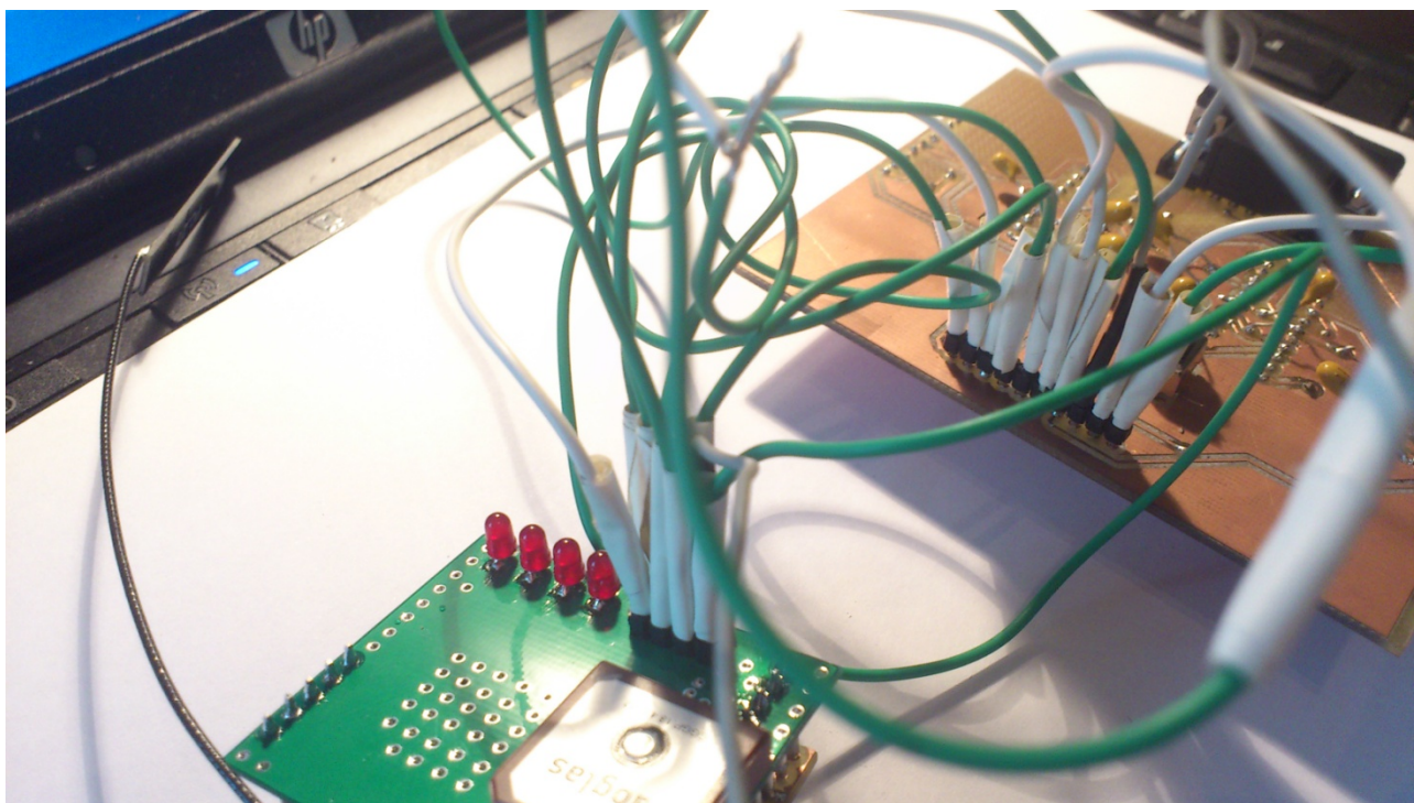
Figura 4.51: Detalle del conexión del dispositivo final de usuario con la placa PC Com.
