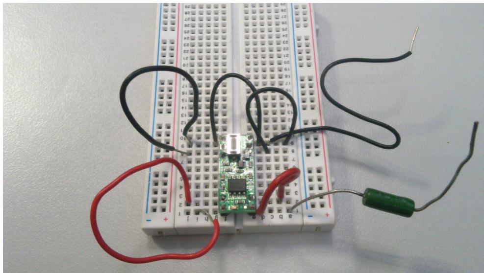
Figura 3.15: Interruptor Pololu con la resistencia conectada a Vin.
